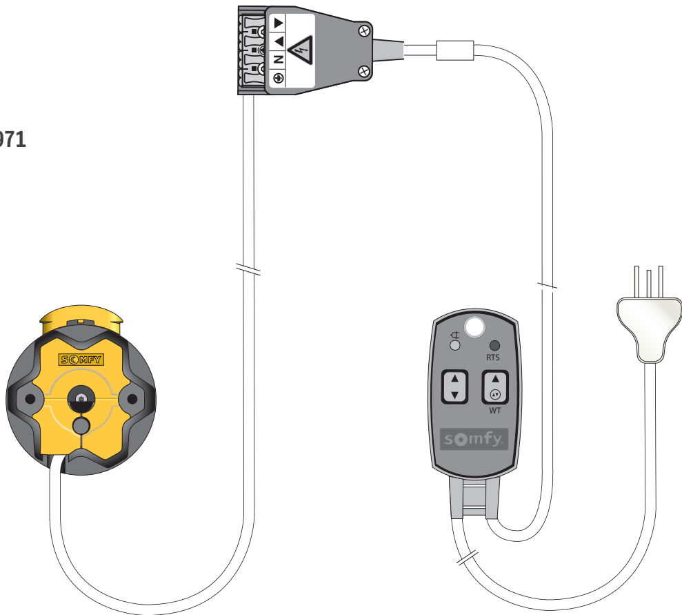
Somfy tubular motor
